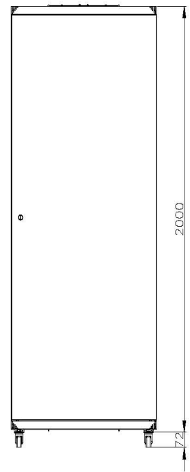
BACK(STEEL DOOR)
